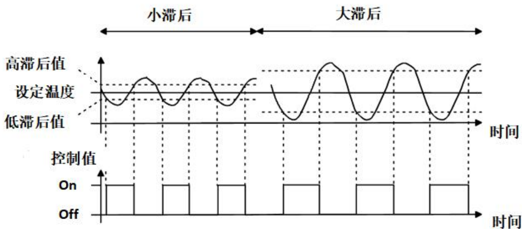
图 5.7.2(2) 两点控制方式下滞后对控制值开关动作的影响 (加热)
