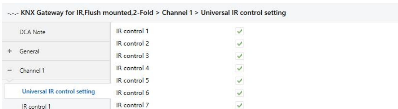
图 5.3.1 (1) “Universal IR control setting” 参数设置界面
