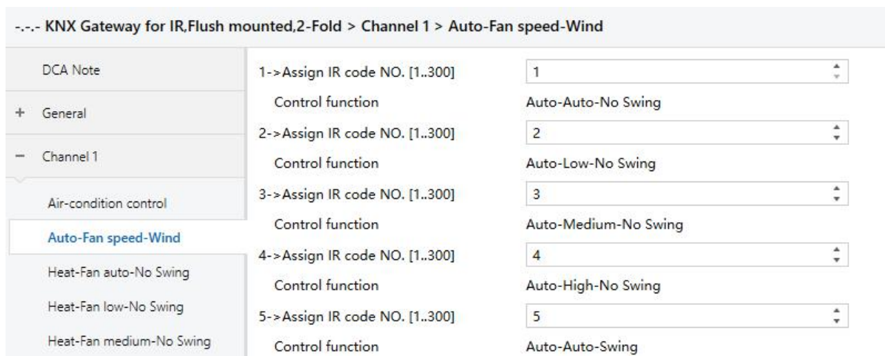
图 5.3.2 (4) “Auto-Fan speed-Wind” 参数设置界面
