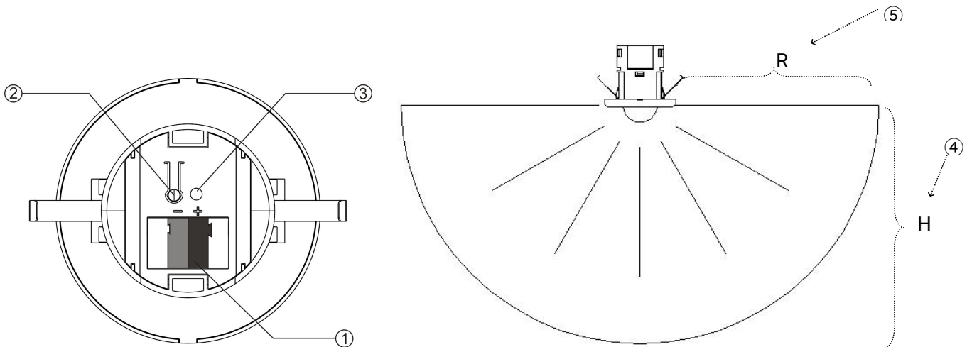
图 3.2(2) 吸顶式红外发射器 V2 (BTIRC-01/00.2)
