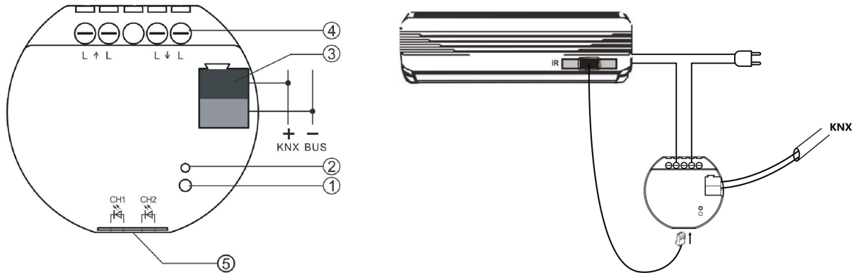
图 3.2(1) 2 路嵌入式红外发射器 (BTIRF-02/00.2)
