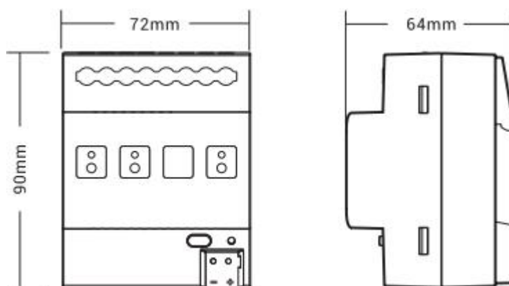
2 路尺寸图
