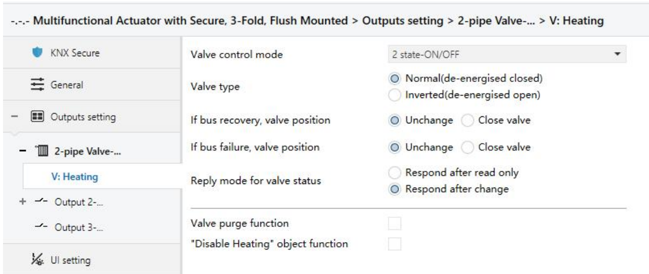
图 4.7.1(1) 参数设置界面“Valve: Heating”
