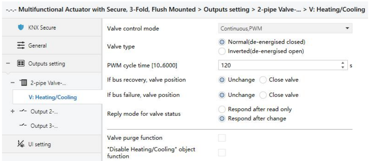
图 4.7.1.2 参数设置界面“Continuous, PWM”
