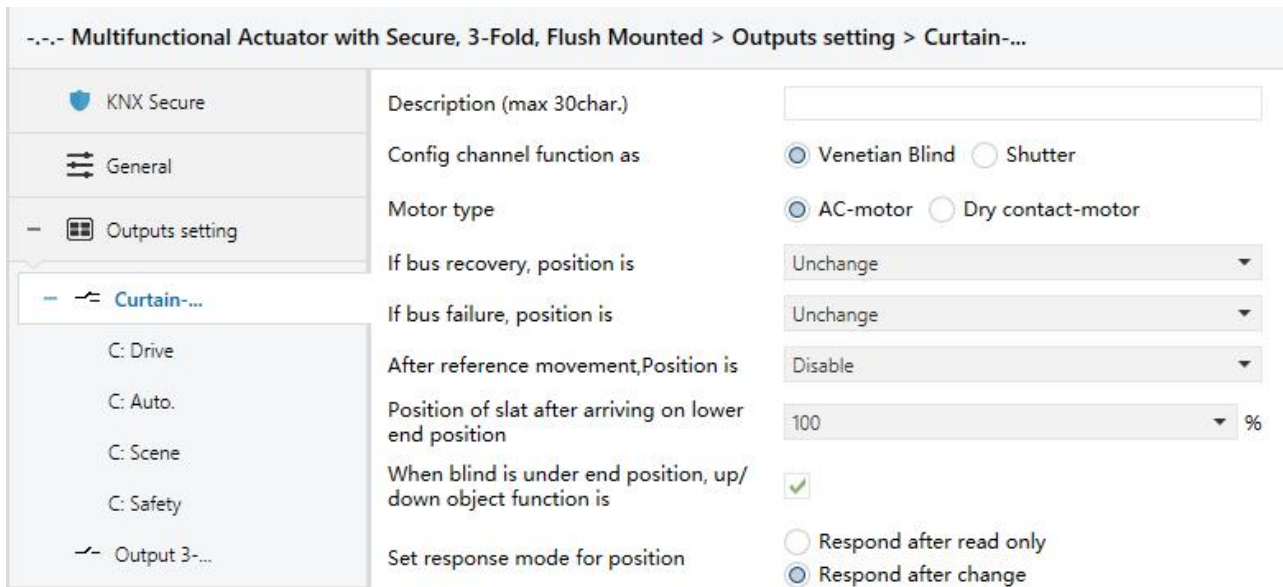
图 4.6.1 参数设置界面 “Output Curtain”
