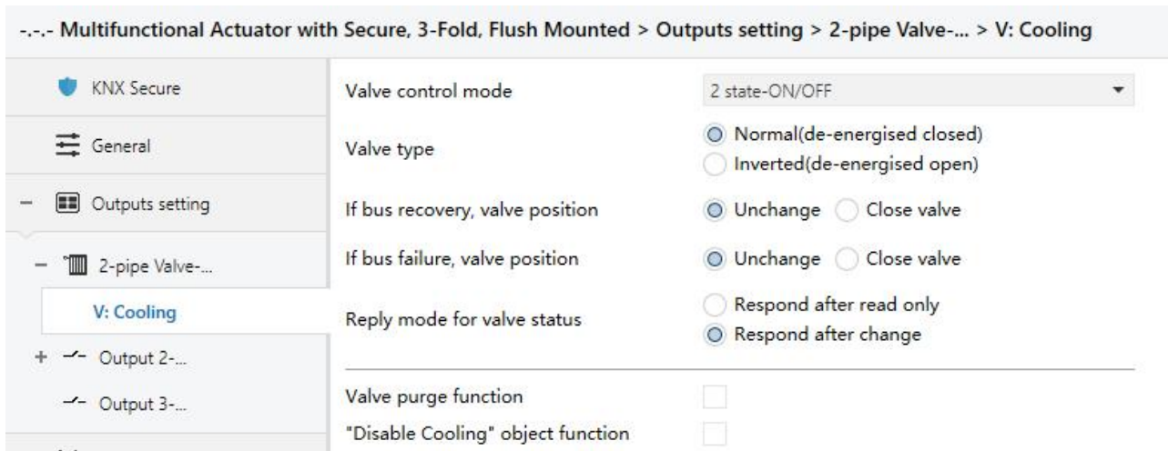
图 4.7.1(2) 参数设置界面“Valve: Cooling”
