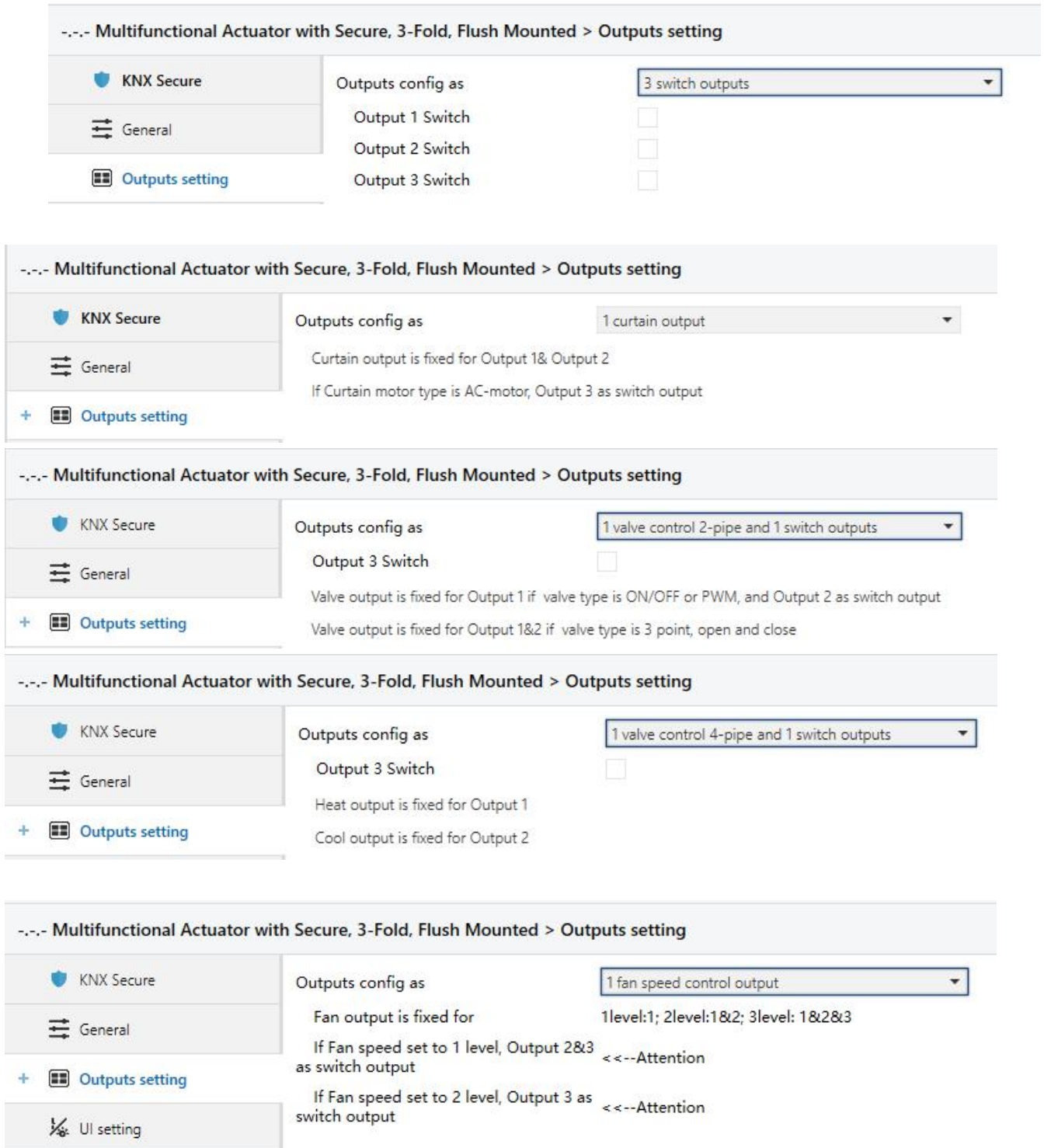
图 4.3 参数设置界面 “Channel configuration”
