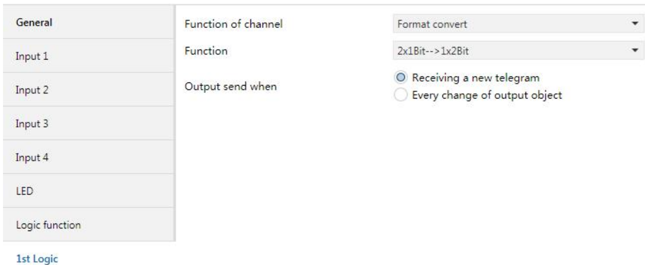
图 4.20 参数设置界面“Logic function – Format convert”
